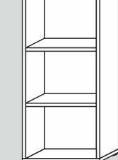
6046/40/F* 46x102x40cm (BxHxT) 6046/32/F* 46x102x32cm (BxHxT)
