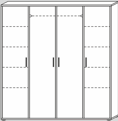
60823/F/G* 178x182x56cm (BxHxT)
