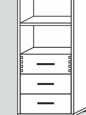
6049/40/F/G* 46x102x40cm (BxHxT) 6049/32/F/G* 46x102x32cm (BxHxT)
