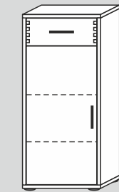
6054L/40/F/G* 46x102x40cm (BxHxT) 6054L/32/F/G* 46x102x32cm (BxHxT)
