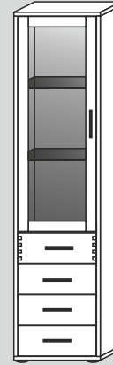
60714L/40/F/G* 46x182x40cm (BxHxT) 60714L/32/F/G* 46x182x32cm (BxHxT)
