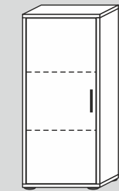
6052L/40/F/G* 46x102x40cm (BxHxT) 6052L/32/F/G* 46x102x32cm (BxHxT)
