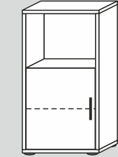
6036L/40/F/G* 46x86x40cm (BxHxT) 6036L/32/F/G* 46x86x32cm (BxHxT)
